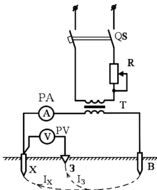
Рисунок 1 – Схема измерений методом «амперметра – вольтметра»
