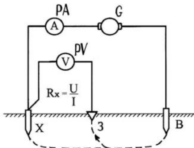
Рисунок 3 - Принципиальная схема измерения сопротивления растеканию тока заземления R_x по методу «амперметра-вольтметра»
