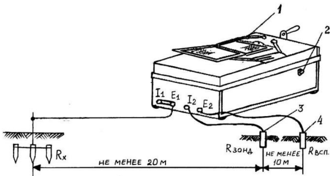
Рисунок 4 – Принципиальная схема включения измерителя заземления типа МС – 0,8 (трехпроводная схема, большие сопротивления):
