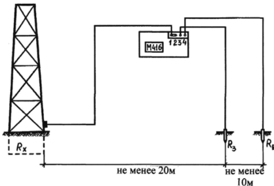
Рисунок 9 – Трёхпроводная схема подключения М 416 по трем зажимам
