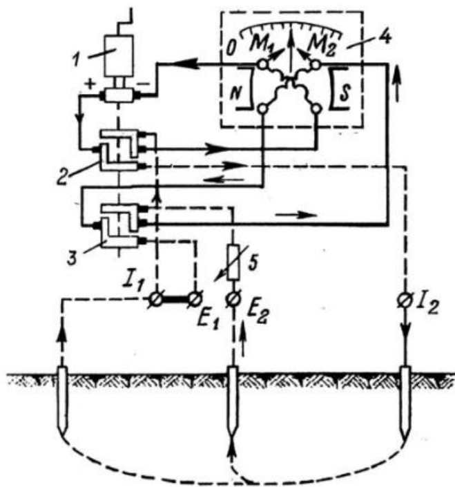
Рисунок 2 - Схема измерителя заземления типа МС-08, где: 1 – генератор постоянного тока; 2 – прерыватель тока; 3 – выпрямитель; 4 – логометр; 5 - регулируемое сопротивление.
