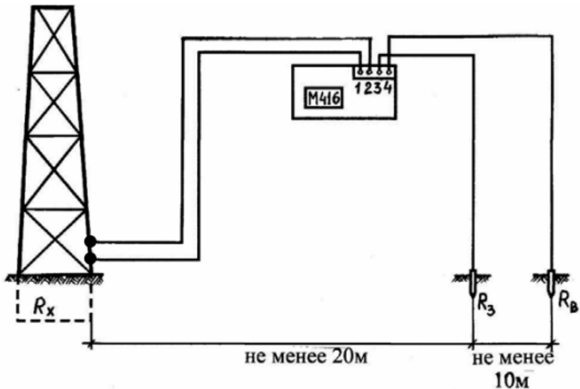
Рисунок 10 - Четырехпроводная схема подключения М 416 по четырем зажимам
