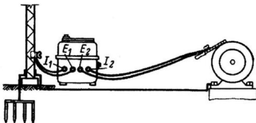
Рисунок 7 - Измерение сопротивления заземляющей проводки измерителем МС-08 при больших расстояниях между испытываемым оборудованием и магистралью
