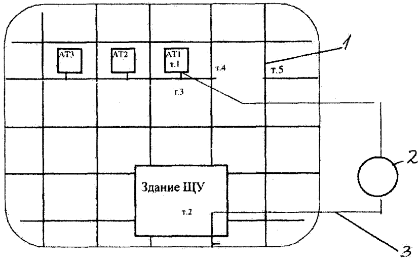
Рис. П2.1. Схема прокладки магистралей ЗУ: 1 - магистраль заземления; 2 - ИППТ; 3 - соединительные провода
