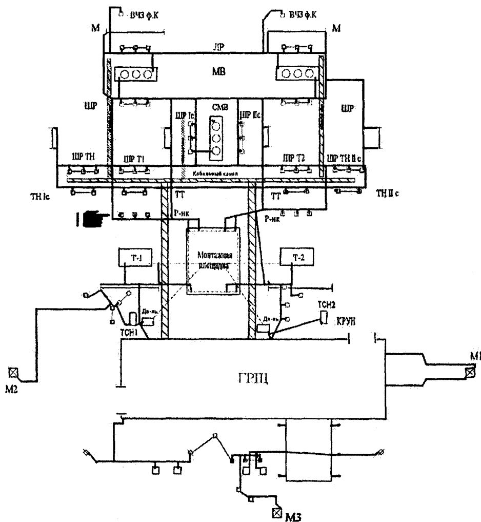
Рис. 1. Схема-план заземляющего устройства подстанции:
