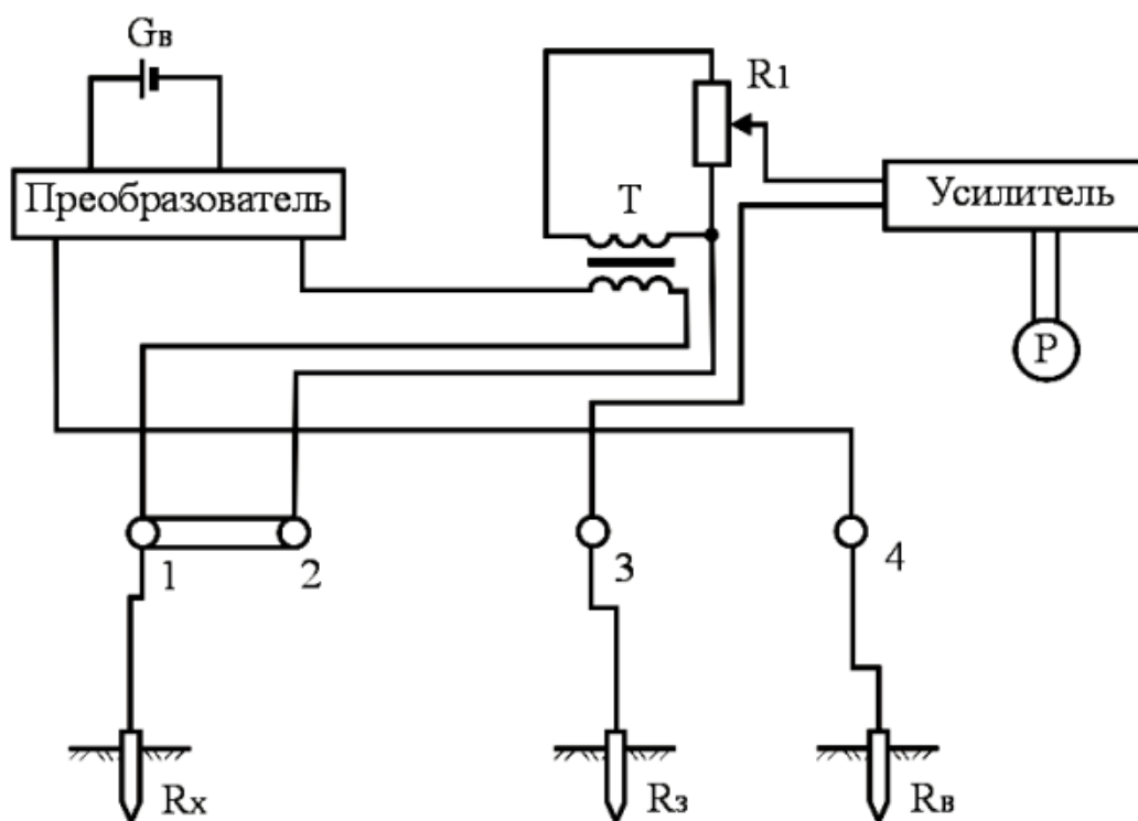
Рисунок 8 - Структурная схема измерителя заземления М 416
