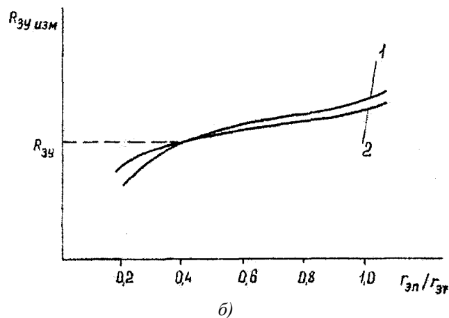
Рис. 3. Зависимость измеренного сопротивления от расстояния потенциального электрода до токового: а - при достаточном удалении токового электрода; б - при недостаточном удалении токового электрода; 1 - кривая при r_{эт} = 3Д ; 2 - кривая при r_{эт} = 2Д
