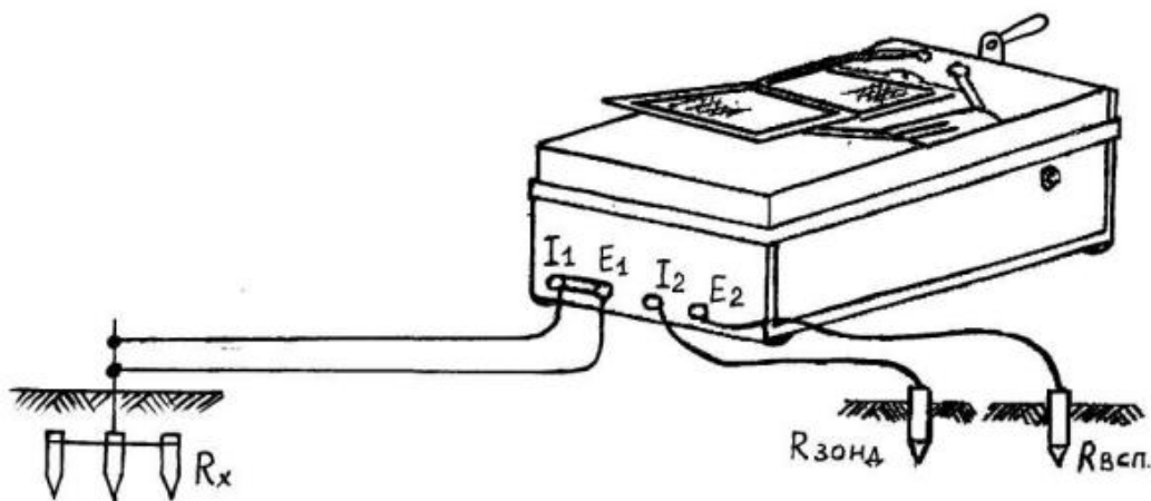
Рисунок 5- Схема измерения сопротивления заземлителей измерителем заземления МС – 0,8 (четырёхпроводная схема – малые сопротивления)
